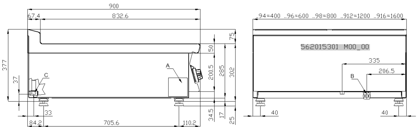
FIG. 2 BMT...
